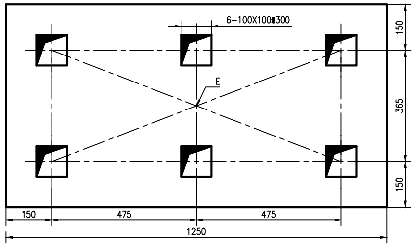
风机基础平面示意图
